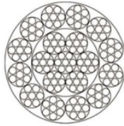
18x7+IWRC
