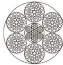
6X36SW+IWRC
