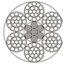
6X19+IWRC
