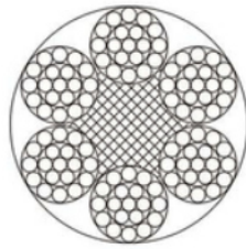
6X19+FC
